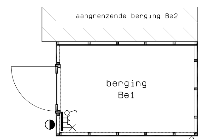
plattegrond
