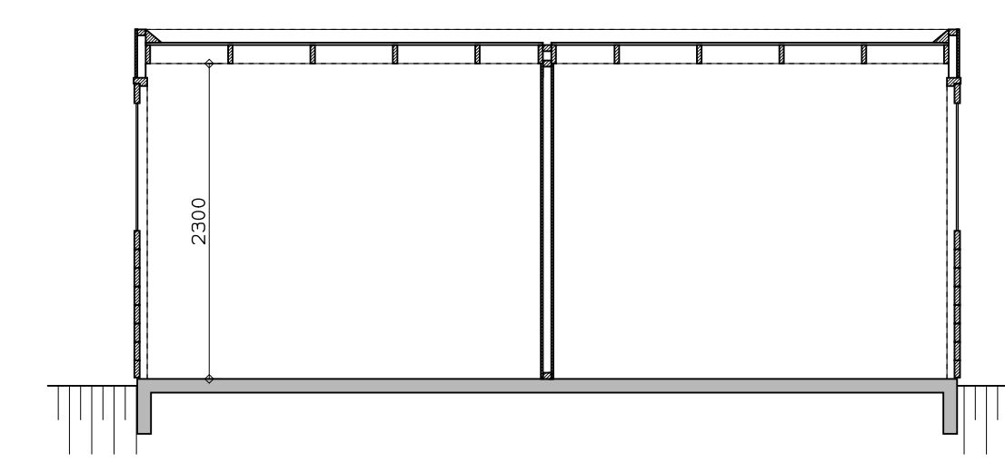
doorsnede
