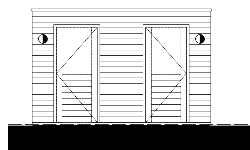
voorgevel
